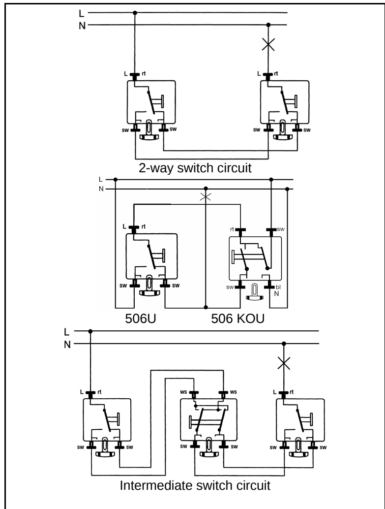
Wiring diagrams 506 U
